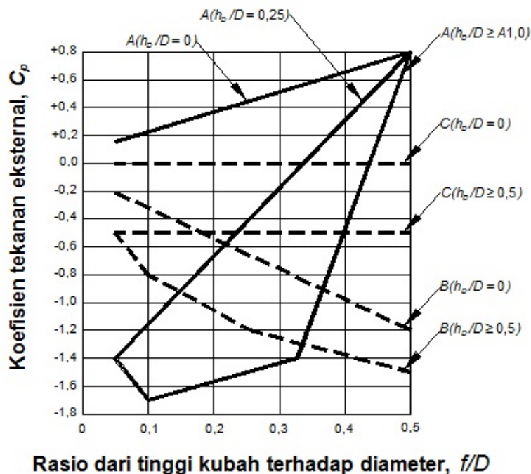
Koefisien tekanan eksternal untuk kubah dengan dasar lingkaran
