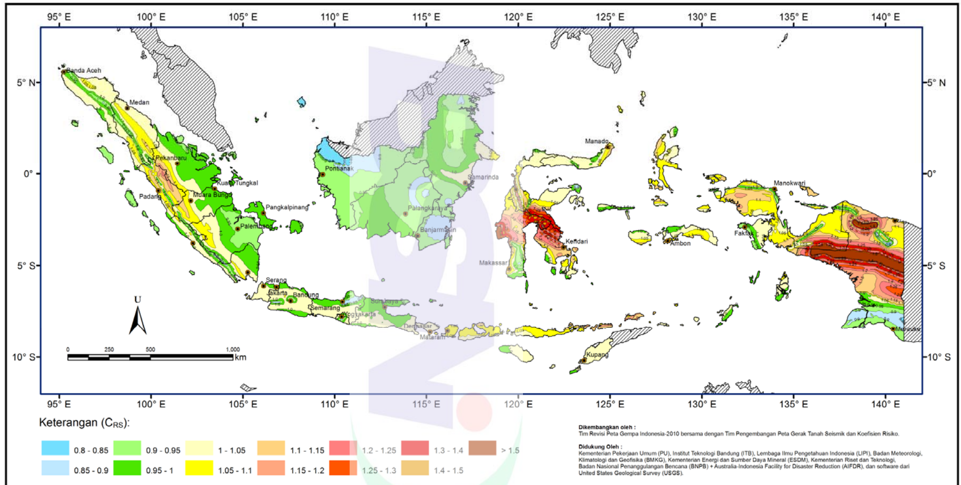
Gambar 12 - C_{RS} , Koefisien risiko terpetakan, periode respons spektral 0,2 detik
