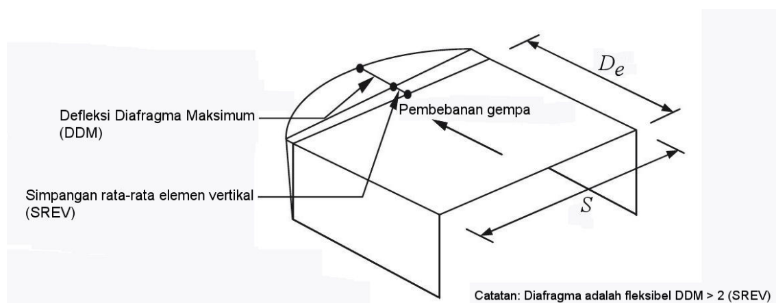
Gambar 3 - Diafragma fleksibel
