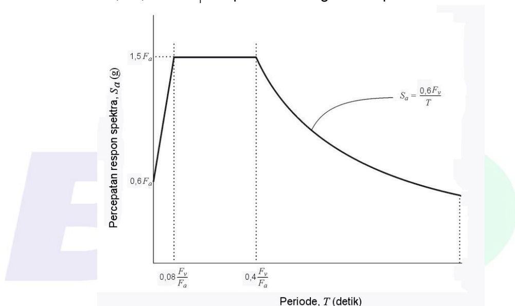
Gambar 2 - Batas Bawah Spektrum Respons MCE_R Deterministik
